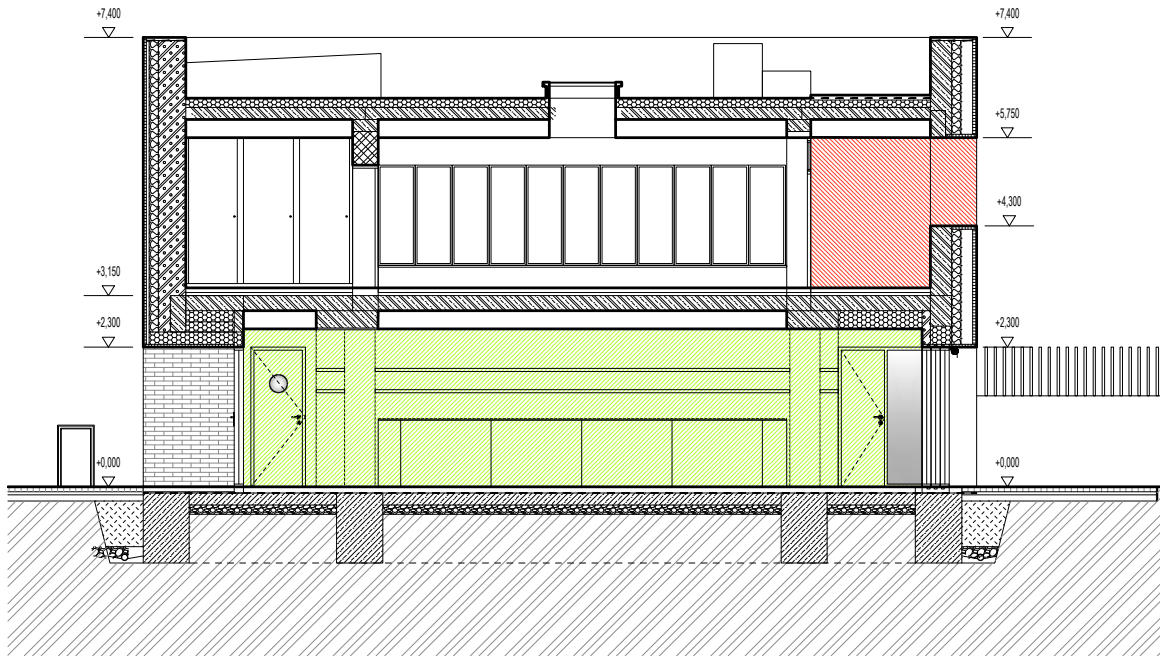
ŘEZ C
